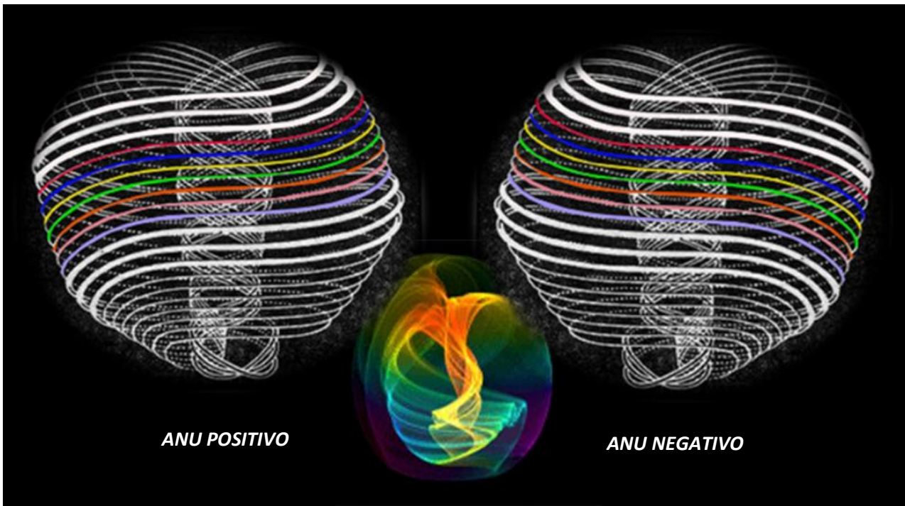
FIGURA 6. COPPIE DI ANU CON DIECI VORTICI
